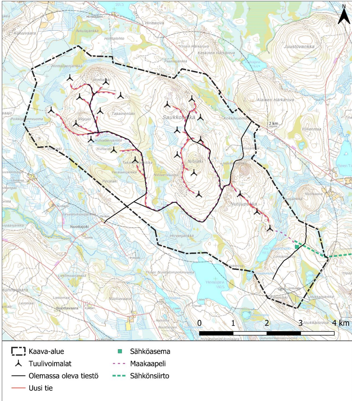
Kuva 3.2. Voimalasijoittelu ja huoltotiestö, sähköasema sekä sähkösiiro.
